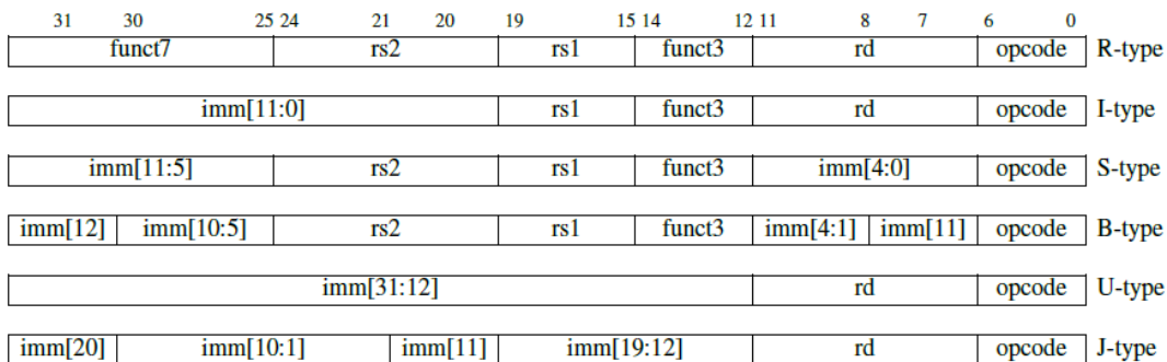
图 2.2: RISC-V 指令格式。我们用生成的立即数值中的位置（而不是通常的指令立即数域中的位置）(imm[x])标记每个立即数子域。第十章解释了控制状态寄存器指令使用 I 型格式的稍微不同的做法。（本图基于 Waterman 和 Asanovi'c 2017 的图 2.2）。
