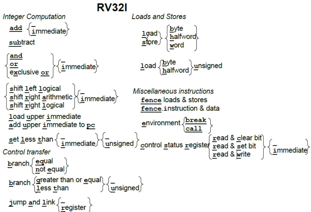
图 2.1: RV32I 指令图示。把带下划线的字母从左到右连接就组成了 RV32I 指令。花括号 {} 表示集合中垂直方向上的每个项目都是指令的不同变体。集合中的下划线_意味着不包含这个字母的也是一个指令名称。例如，左上角附近的符号表示以下六个指令：and, or, xor, andi, ori, xori。
